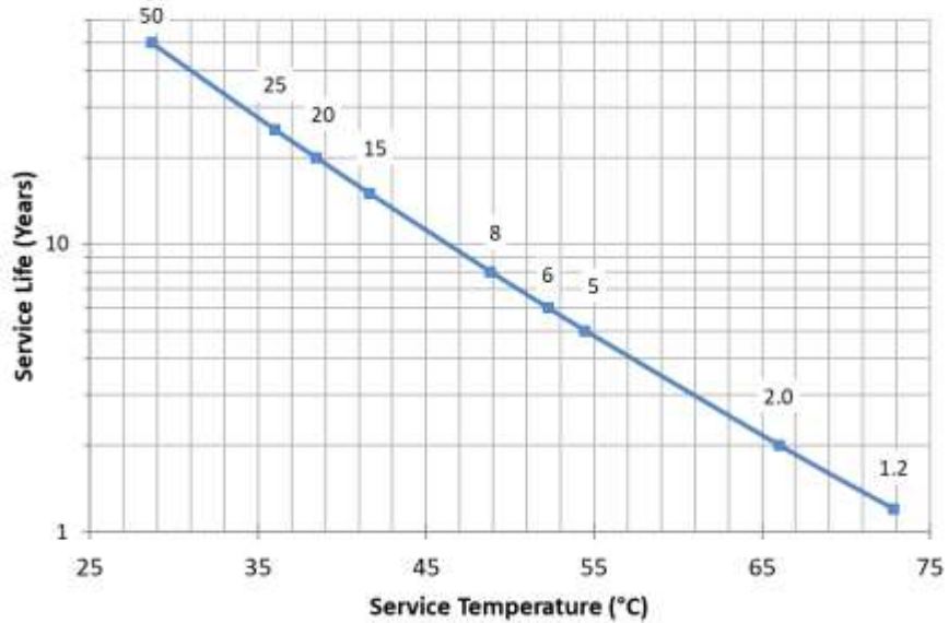
DTN2070 Service Life vs. Temperature (°C)
